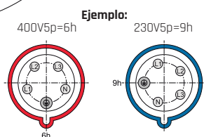
Vista frontal de la clavija o conector
